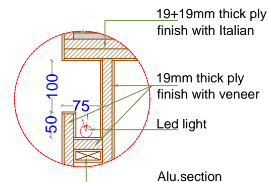
Detail D3
