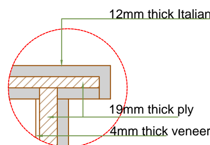
Detail D2
